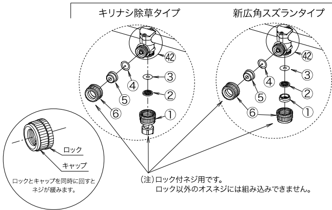
Ⓐ 15型噴口噴管部詳細
