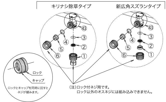
Ⓑ 17型噴口噴管部詳細
