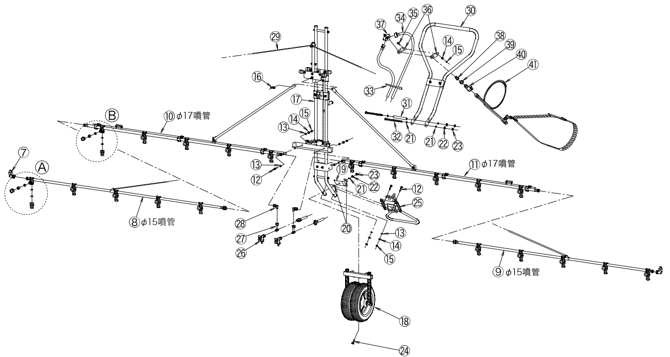
Ⓐ 15型噴口噴管部詳細
