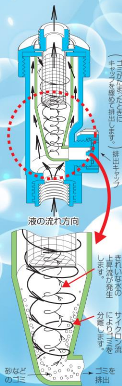
サイクロン流による ゴミ捕集の模式図
