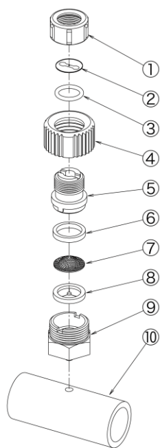
微量ノズル5型
